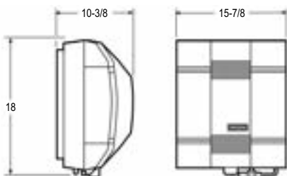
Model: P110-LFP1518
